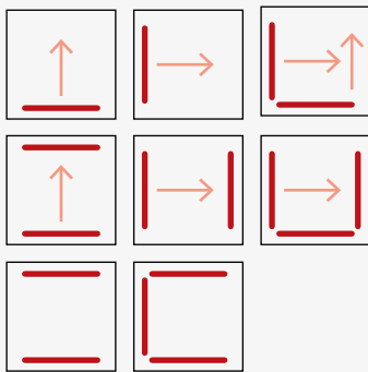
Différentes dispositions des barres de soudure
