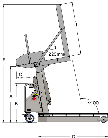
VERSION BSMBRLT Hauteur de déversement A = 1270mm
