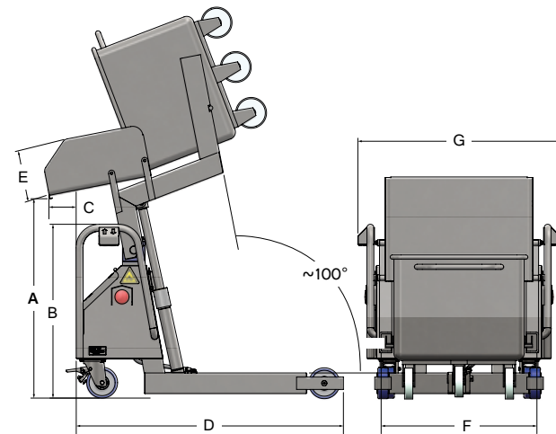
VERSION BSMBR Hauteur de déversement A = 970mm
