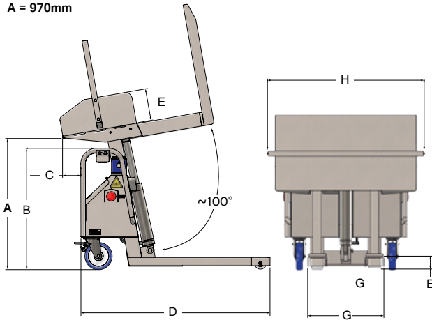
VERSION BSMST Hauteur de déversement A = 970mm
